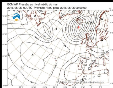
Figura 1 – Carta sinótica.
